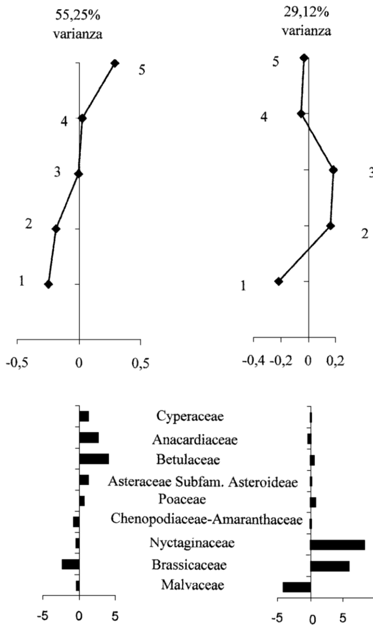
Lám. 3. Diagramas del Análisis de Correspondencia de las muestras (arriba) y los taxa (abajo) del perfil Taritolay.
